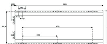
CONVERTISSEUR CHARGEUR 24Vdc/230Vac 24Vdc/230Vac INVERTER CHARGER
