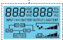
CONVERTISSEUR CHARGEUR 24Vdc/230Vac 24Vdc/230Vac INVERTER CHARGER
