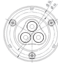
Montage avant Front mounting
